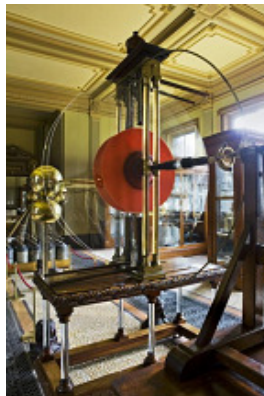
KH elektriseer machine
